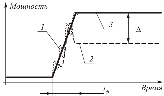
Рис. 5. Иллюстрация искажений формы цифрового импульса действием многолучевой интерференции. На рисунке обозначено: t_{\phi} – длительность фронта реального трапециoidalного импульса, 1 и 2 – искажённые импульсы, 1 – интерферометр к моменту окончания t_{\phi} остался в районе прежней рабочей точки, 2 – положение рабочей точки интерферометра изменилось, появилась отражённая волна с амплитудой \Delta ; 3 – неискажённый импульс
