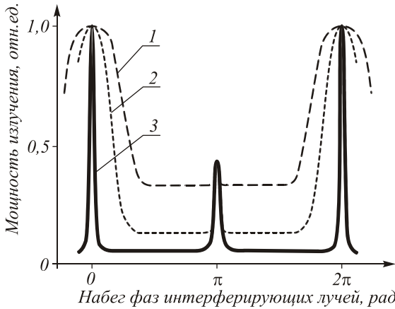
Рис. 3. Иллюстрация зависимости передаточной функции многолучевого интерферометра от набега фаз interfering лучей для различных значений \rho : 1 – \rho_{\text{ИФП}} = 0,6 ; 2 – \rho_{\text{ИФП}} = 0,8 ; 3 – двухрезонаторный многолучевой интерферометр с коэффициентом отражения – \rho_{\text{ДИФП}} = 0,8 . [13]
