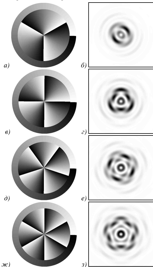
Рис. 6. Фазовые функции ДОО для формирования суперпозиций оптических вихрей с разницей номеров порядков 2, 3, 4, 5 соответственно (а, в, д, ж), распределение интенсивности в сформированных ими пучках (б, г, е, з)
