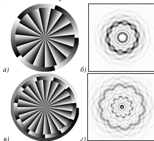
Рис. 11. Фазовые функции ДОО для формирования суперпозиций оптических вихрей 5-го и 15-го соответственно (а), суперпозиции 1-го, 11-го и 21-го порядков (в), распределение интенсивности в сформированных ими пучках (б, г)
