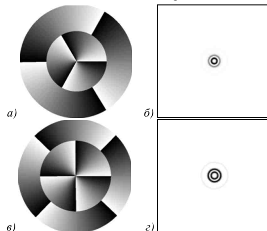
Рис. 2. ДОЭ и соответствующие им световые кольца с равными энергиями (а, б) и равными яркостями (в, г)
