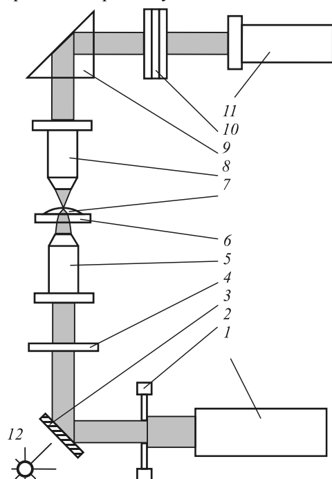
Рис. 16. Оптическая схема установки по вращению агломерации микрочастиц в сложном вихревом пучке.
