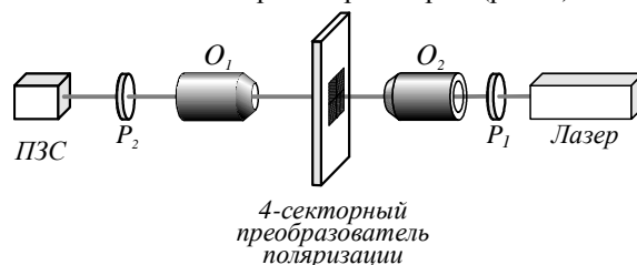
Рис. 5. Схема эксперимента: Laser – He-Ne лазер, P 1 и P 2 – линейные поляризаторы, O 1 – объектив 40 ×, O 2 – объектив 10 ×
