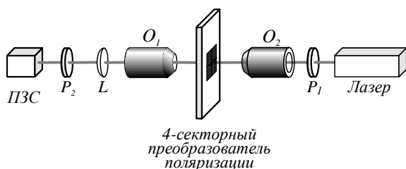
Рис. 7. Схема эксперимента: Laser – He-Ne – лазер, P_1 и P_2 – линейные поляризаторы, O_2 – объектив 40\times , O_1 – объектив 10\times , L – линза (с фокусным расстоянием 24 мм)
