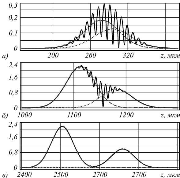
Рис. 2. Амплитуда импульсов для TE-мод волновода (1,1) (точечная линия), (1,3) (пунктирная линия) и их суперпозиции (сплошная линия) в различные моменты времени: t = 2 нс (а), t = 5 нс (б), t = 10 нс (в)
